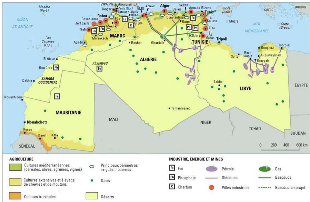
Fig.1.2. Répartition des ressources naturelles dans le grand Maghreb
